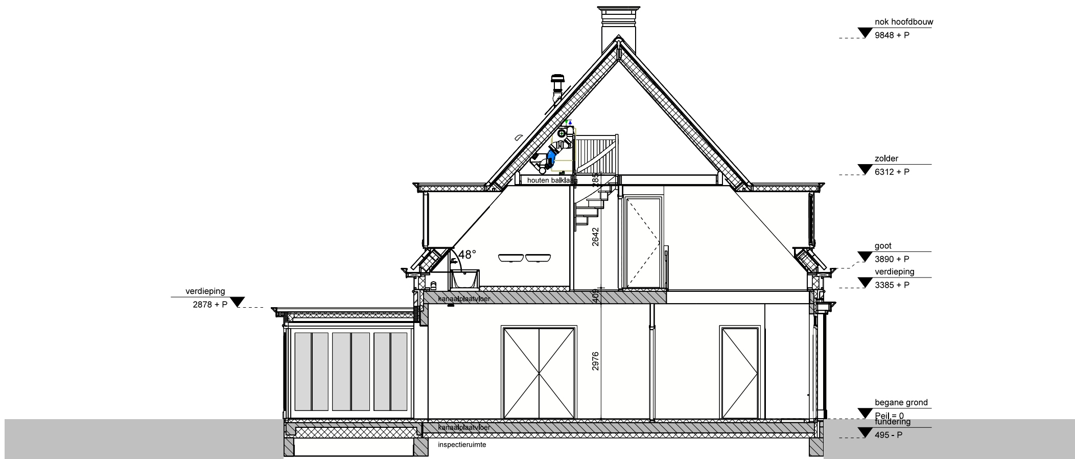
doorsnede B - B
