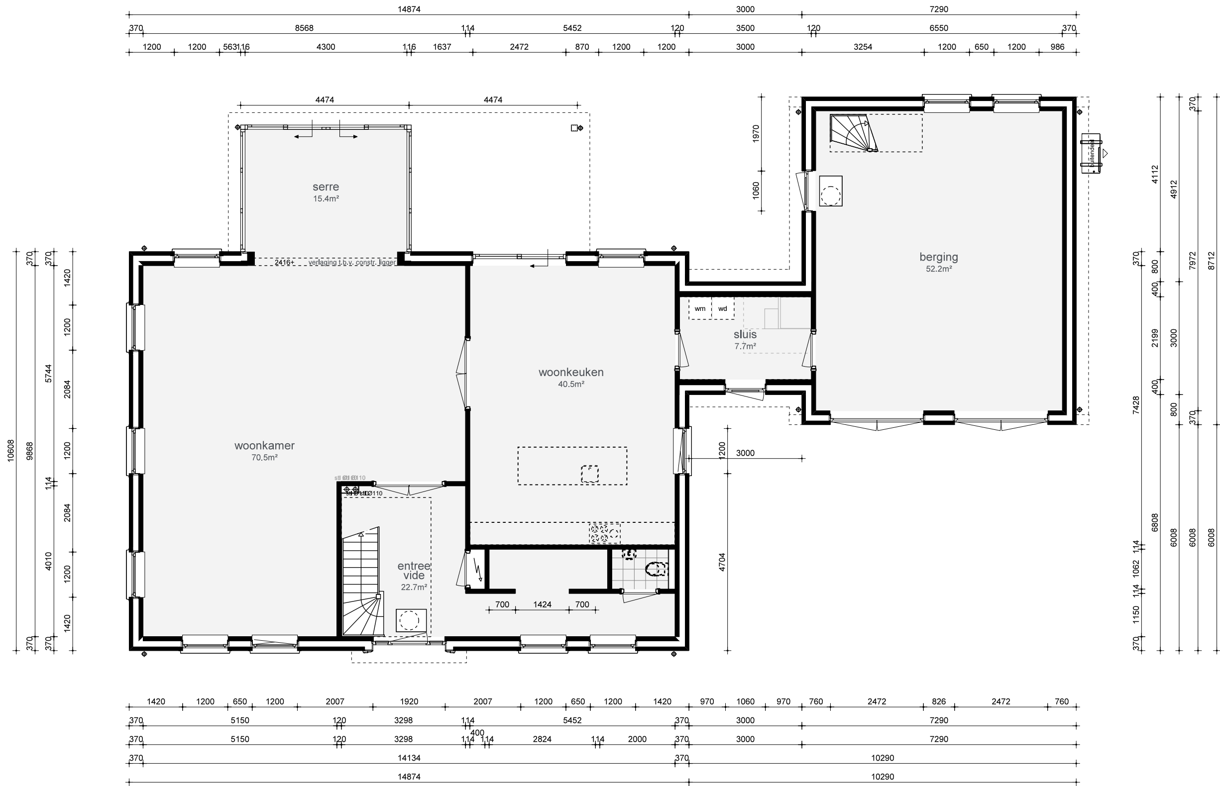
begane grond
